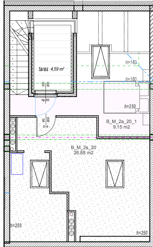
POZIOM GÓRNY antresola
